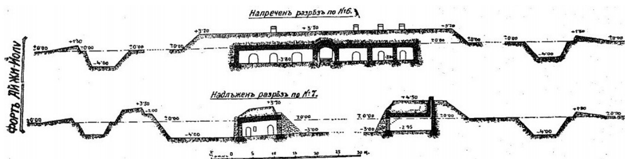
Обр. 2. Скица, показваща напречен и надлъжен разрез на форта Айджийолу. [Дървингов, П. 1931, с. 117].
