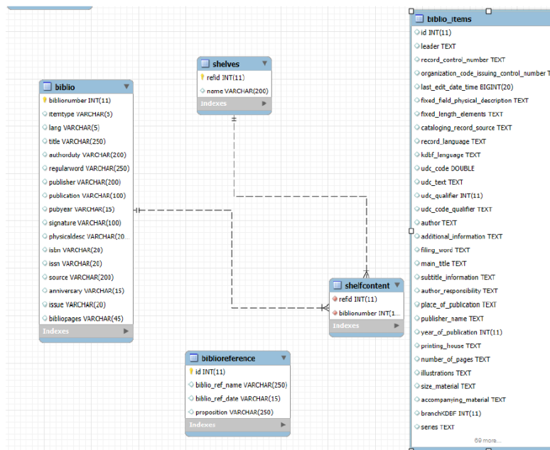
Фигура 2. Реляционна схема на базата от данни
