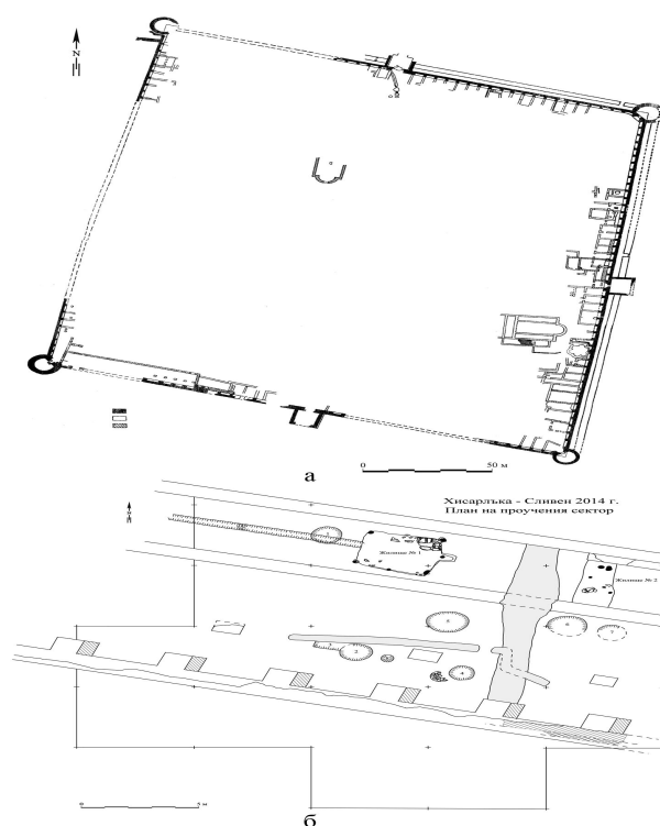
Обр. 1. а – План на крепостта Туида (по Ир. Щерева и др. 2001) б – План на проучената част през 2014 г.
