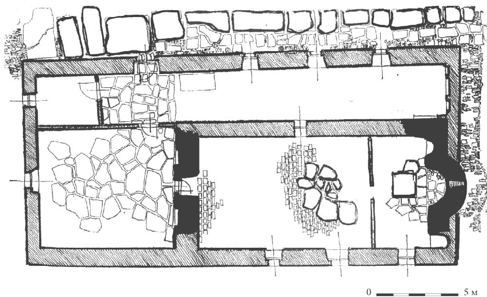
Обр. 1. Църквата “Св. Георги”. План. (по Т. Теофилов).
