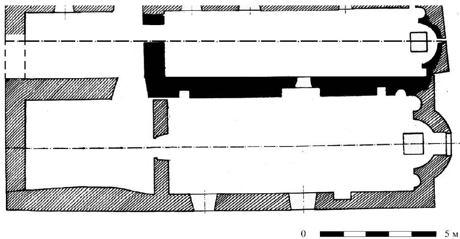
Обр. 2. Храмът “Св. Димитър”. План с маркирани останки от ранната църква “Св. Георги” (по Х. Вачев).
